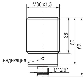
Габаритный чертёж
